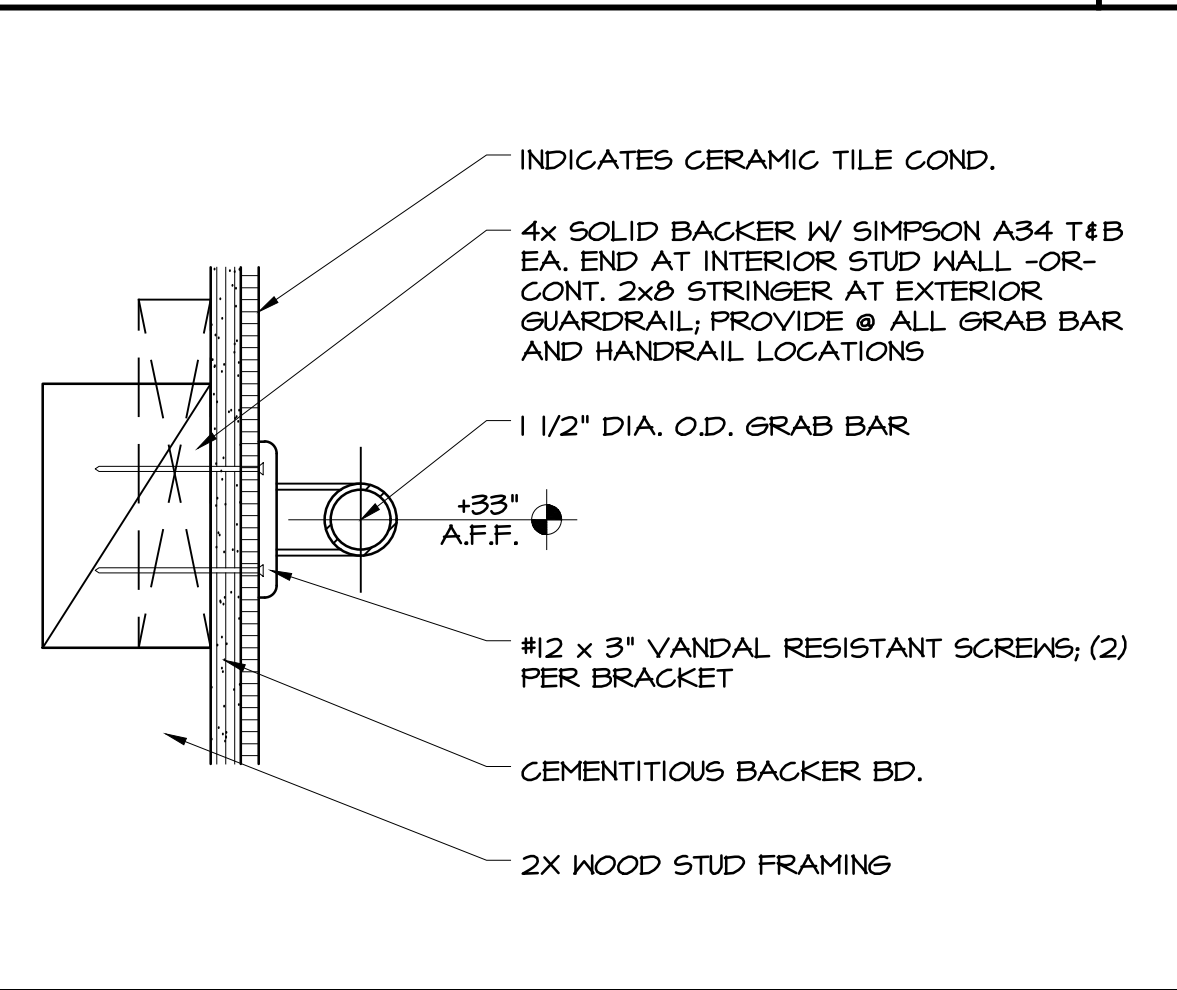
GRAB BAR @ WD. STUD WALL N.T.S. 11
