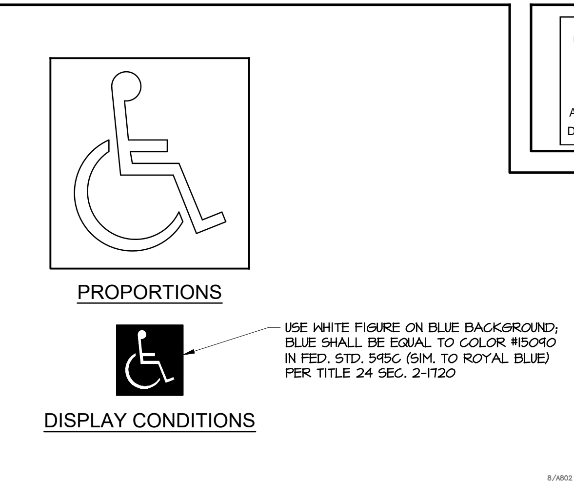
ACCESSIBILITY SYMBOL N.T.S. 1
