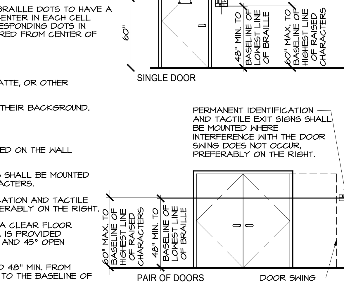
ACCESSIBILITY SIGNAGE N.T.S. 3
