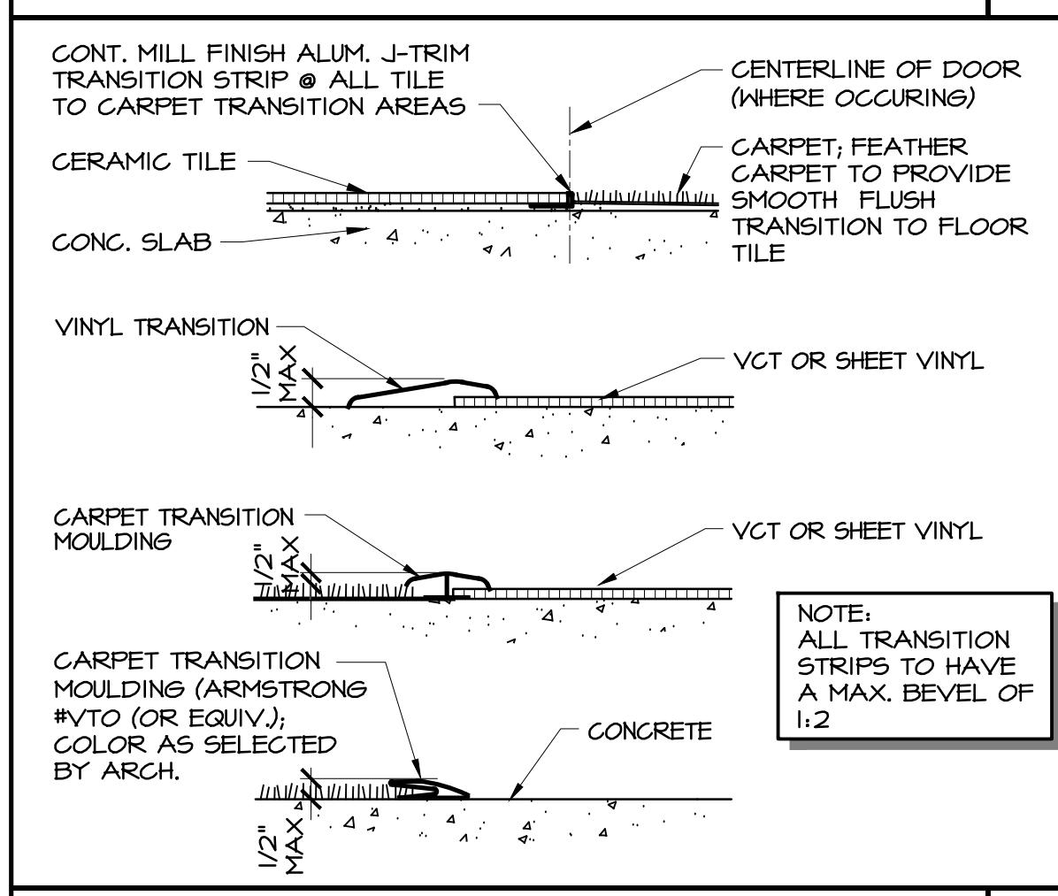
TRANSITION STRIPS N.T.S. 20
