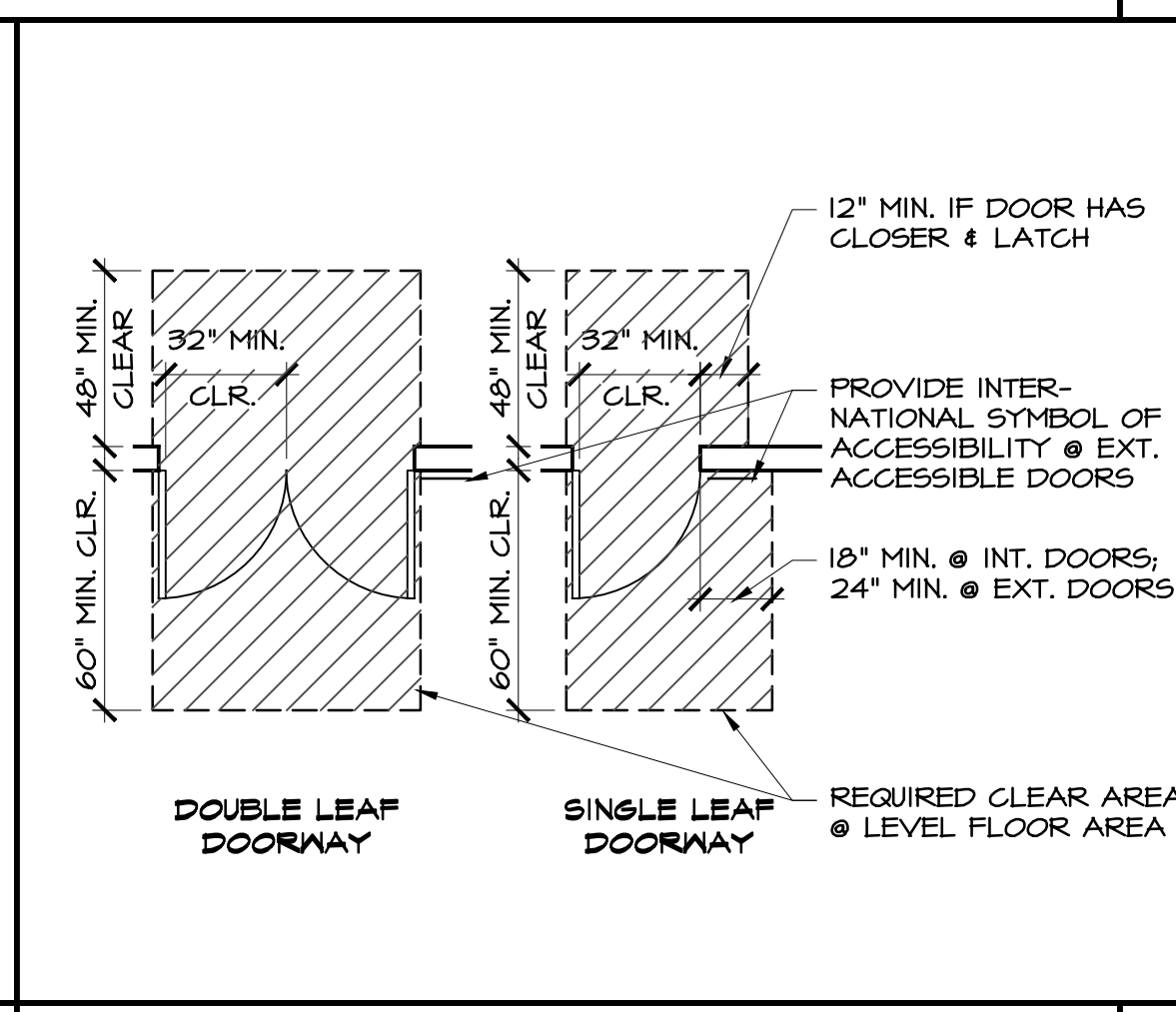
DOORWAY ACCESS N.T.S. 4
